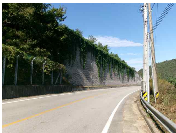
4공구 블럭식 옹벽 04
